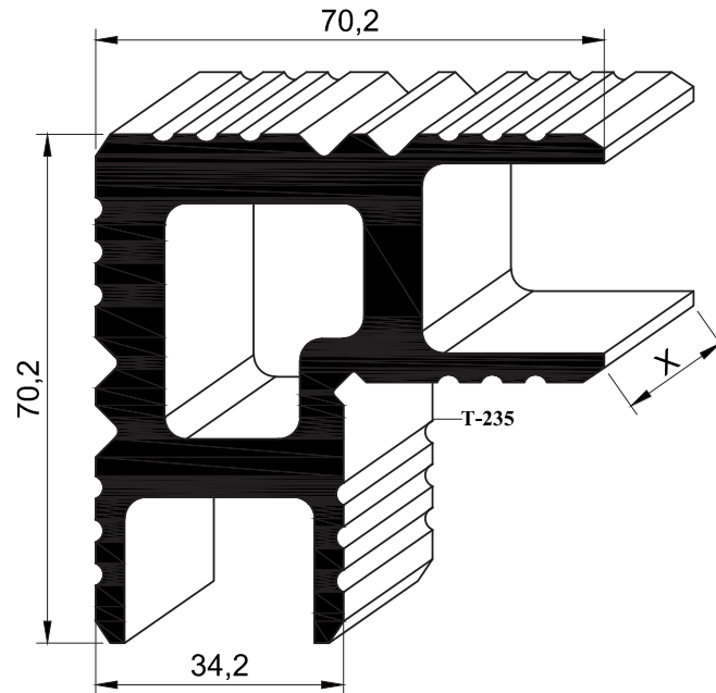
L509 - 4.300 kg/mt
