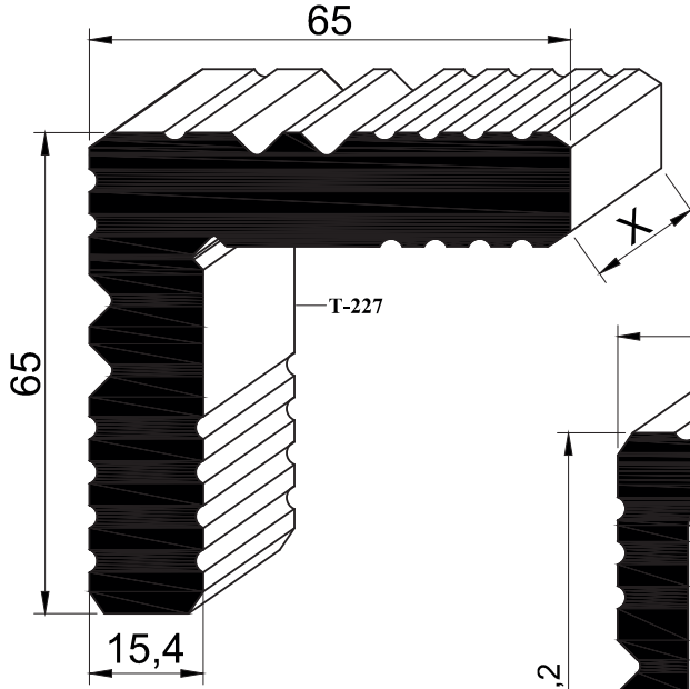
L501 - 4.460 kg/mt
