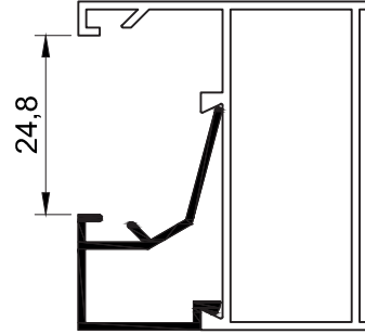
T14 - 0.215 kg/mt
