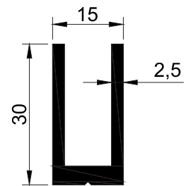
T54 - 0.523 kg/mt
