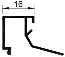
T14 - 0.215 kg/mt
