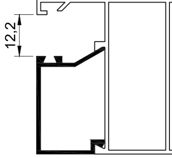
T13 - 0.205 kg/mt
