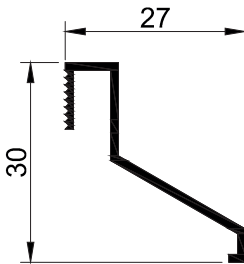
T28 - 0.200 kg/mt
