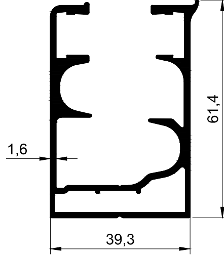
T 2023 - 1.250 kg/m
