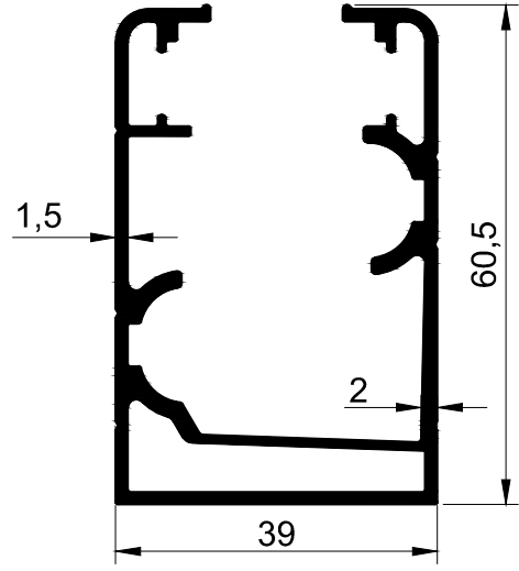
T 2415 - 1.100 kg/m
