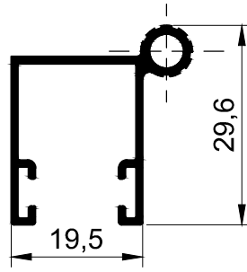
T 1305-0.315 kg/m
