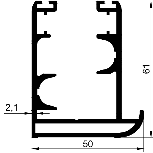
T1073-A - 1.810 kg/m
