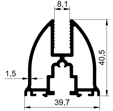
T 2563 - 0.900 kg/m
