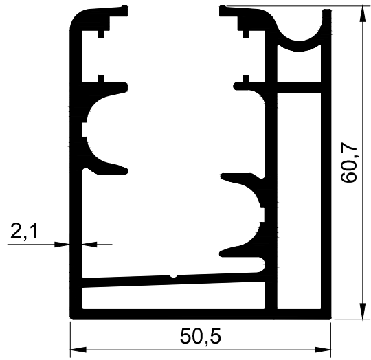
T 876 - 1.887 kg/m
