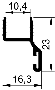
T 589-0.143 kg/m
