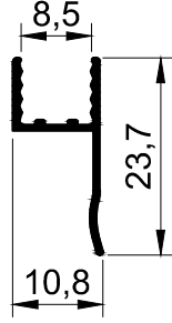
T 938-0.098 kg/m
