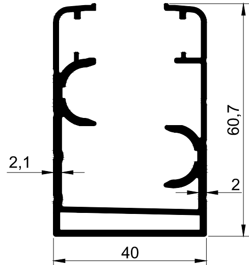
T 2529 - 1.185 kg/m
