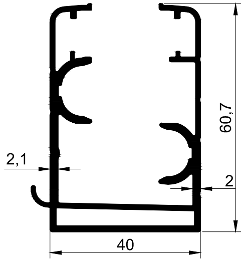
T 2530 - 1.210 kg/m
