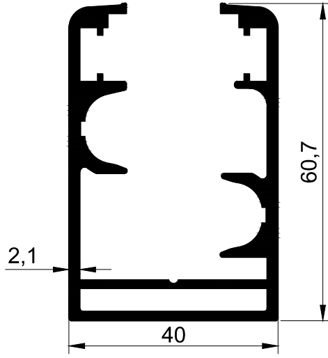
T 2515 - 1.465 kg/m
