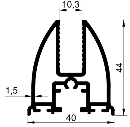
T 2533 0.990 kg/m
