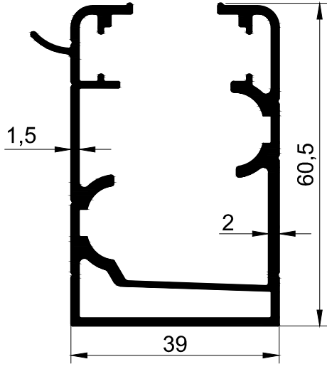
T 2414 - 1.140 kg/m
