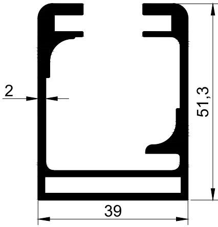
T 2517 - 1.295 kg/m
