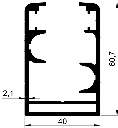
T 2514 1.465 kg/m
