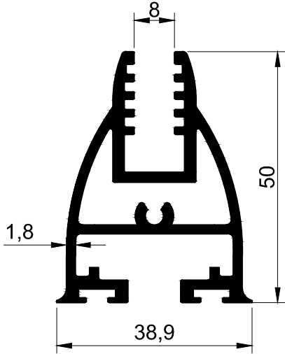
T 2253 - 1.250 kg/m
