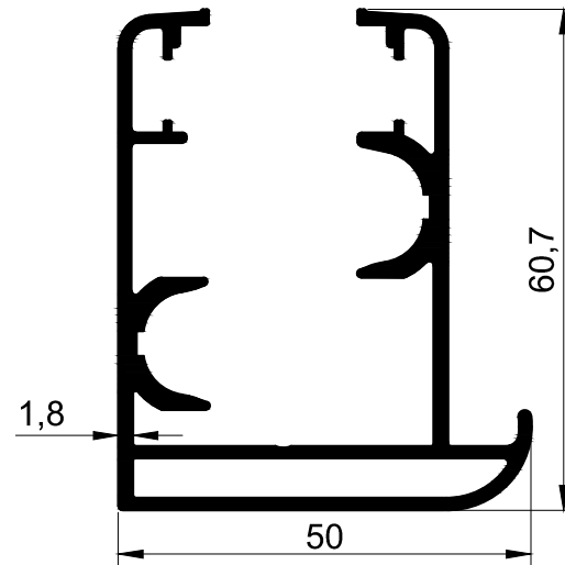
T2522 - 1.352 kg/m
