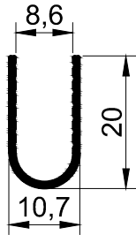
T 2285-0.135 kg/m
