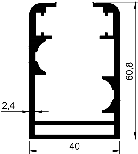
T 2425 - 1.440 kg/m
