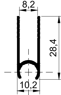
T 1306-0.200 kg/m
