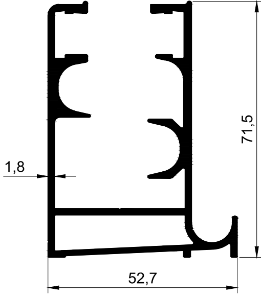
T 2021 - 1.650 kg/m
