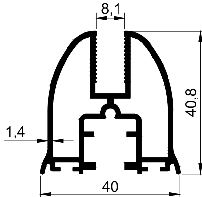
T 2426 - 0.860 kg/m
