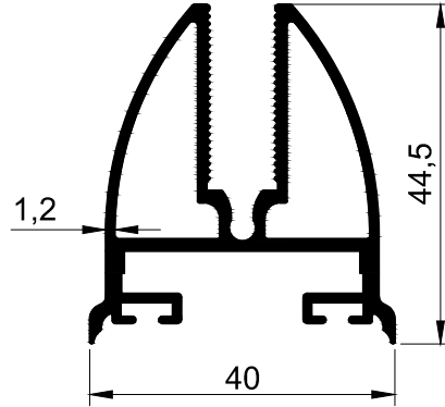
T 2020 0.875 kg/m
