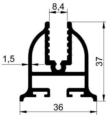
T 2290 - 0.810 kg/m
