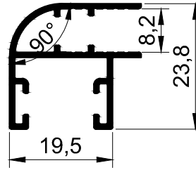
T 839-0.290 kg/m
