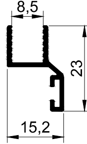
T 916-0.150 kg/m
