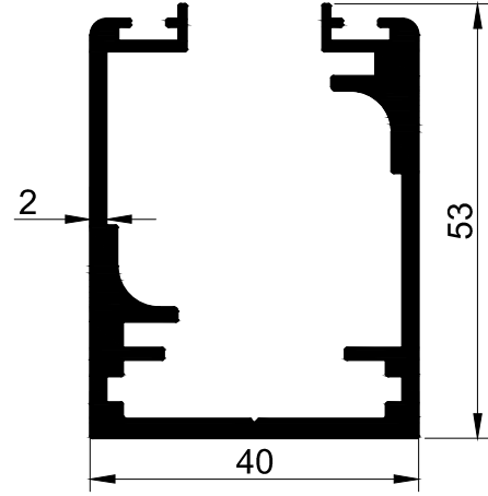
T 2160 - 1.247 kg/m
