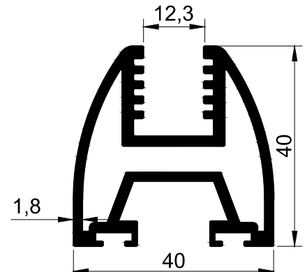
T 2161 - 1.182 kg/m
