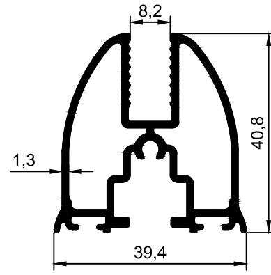
T 2564 0.840 kg/m
