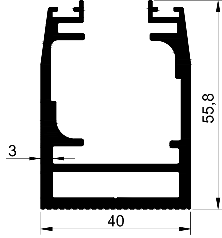
T 2254 - 1.545 kg/m
