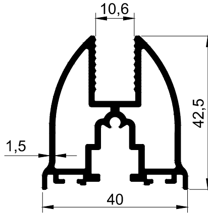
T 2534 0.919kg/m
