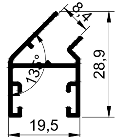
T 840-0.270 kg/m
