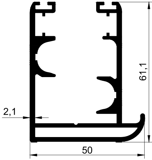
T 1073 - 1.810 kg/m
