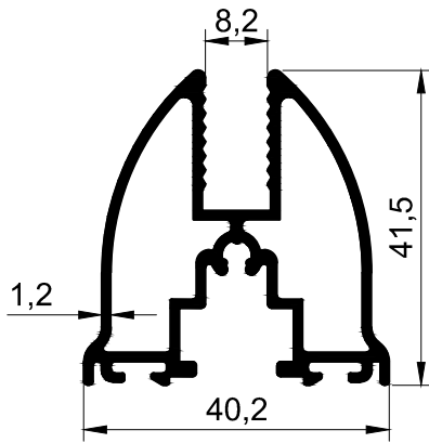
T 2416 0.820 kg/m
