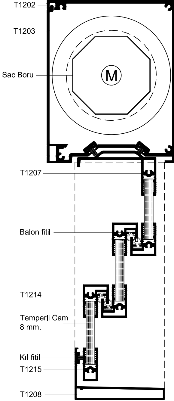
A KESİTİ
