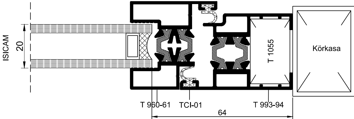
E KESİTİ
