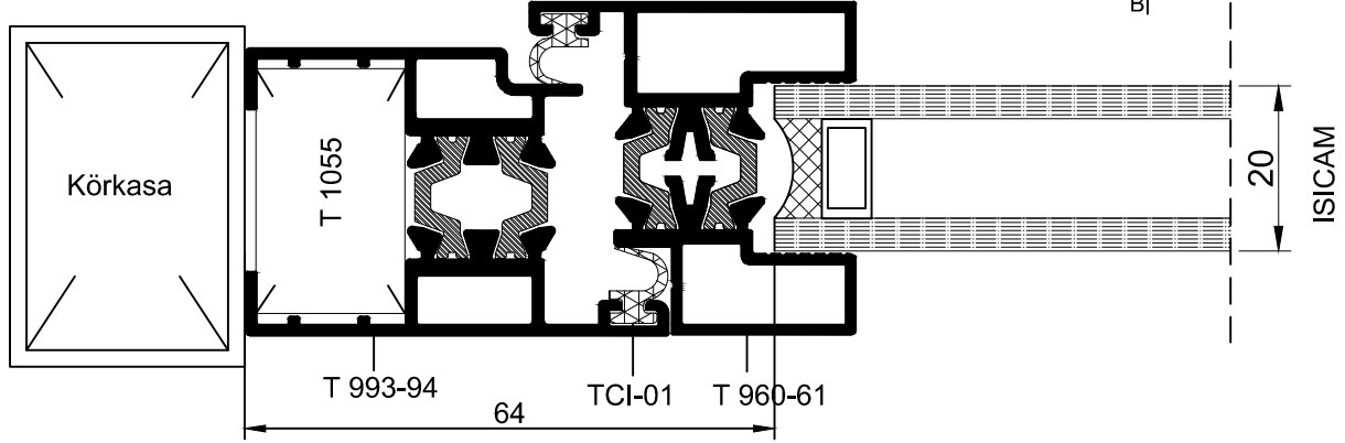
C KESİTİ
