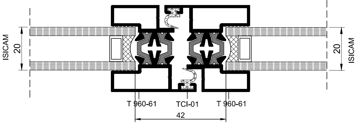
E KESİTİ
