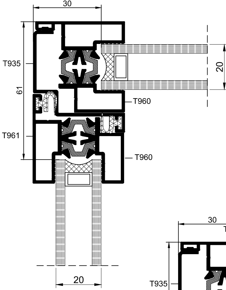
JALUZİLİ CAM BALKON KÖŞE DÖNÜŞ DETAYI
