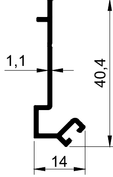
T2397 - 0.210 kg/m Köşe dönüş adaptör profili
