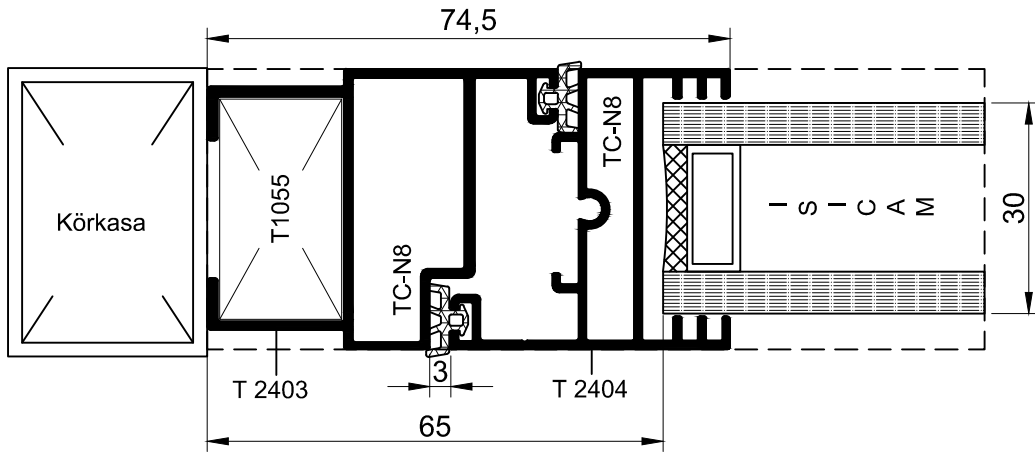
C-KESİTİ
