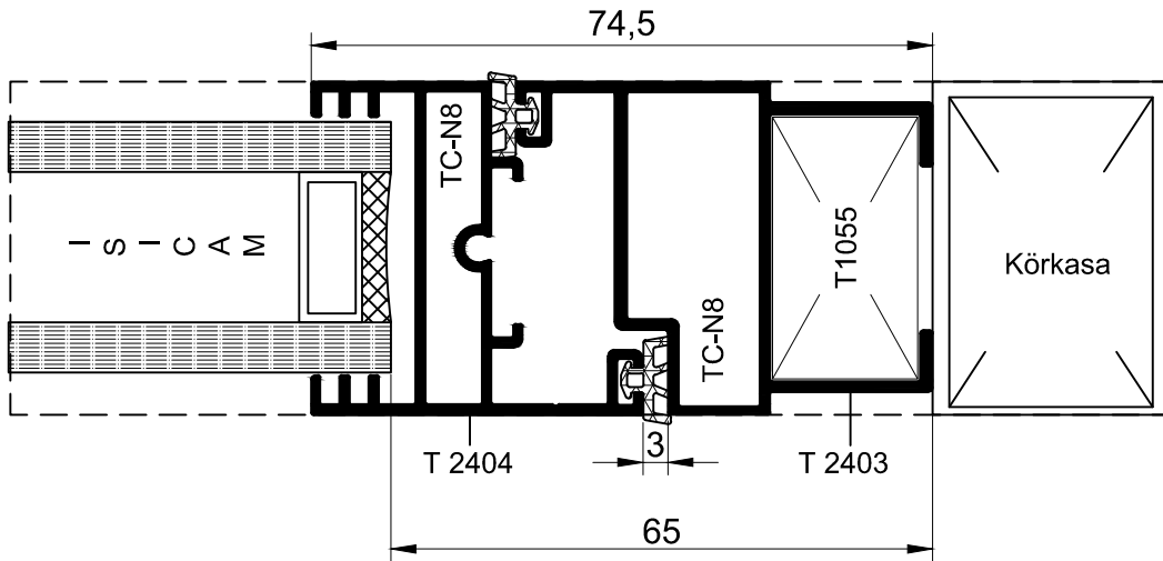
E-KESİTİ
