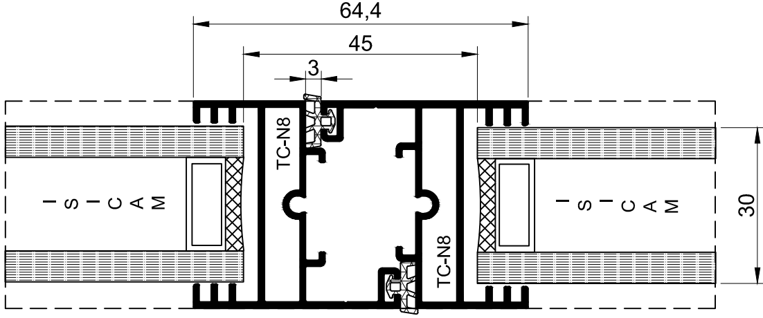
F-KESİTİ
