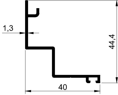
T2447 - 0.336 kg/m Köşe dönüş adaptör profili
