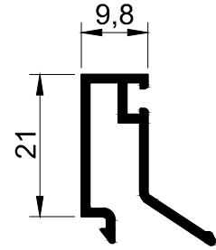
T1046 - 0.230 kg/m
