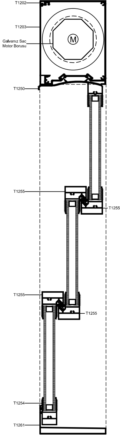
A KESİTİ
