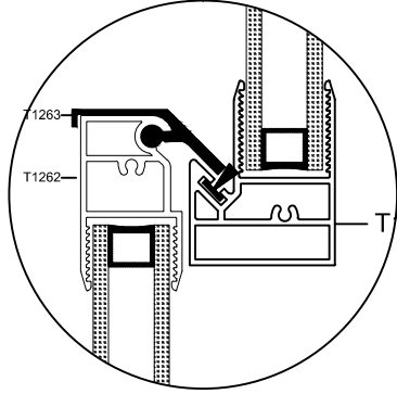
C DETAYI
