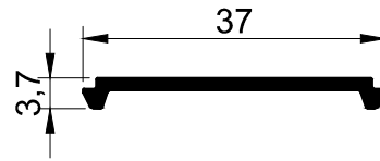
T1256 - 0.169 kg/m
