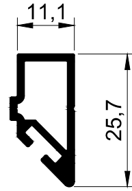
T1260 - 0.277 kg/m
