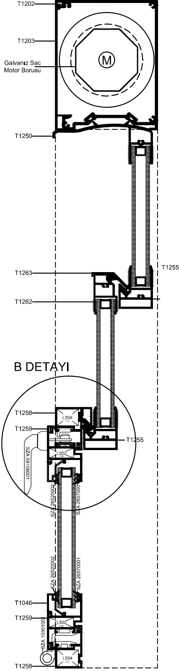
A KESİTİ
