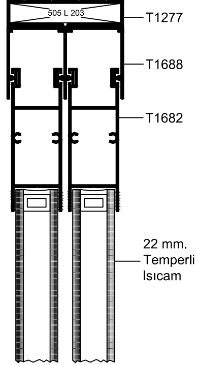
EŞİKLİ SÜRME CAM BALKON
