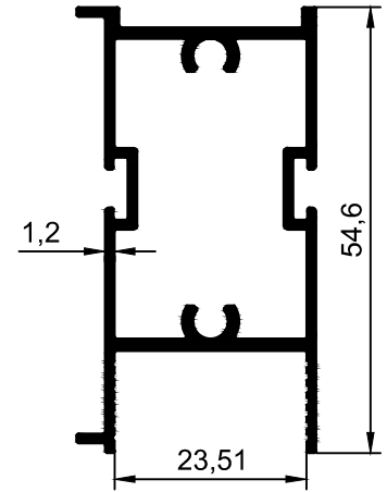
T1685 -0.700 kg/m
