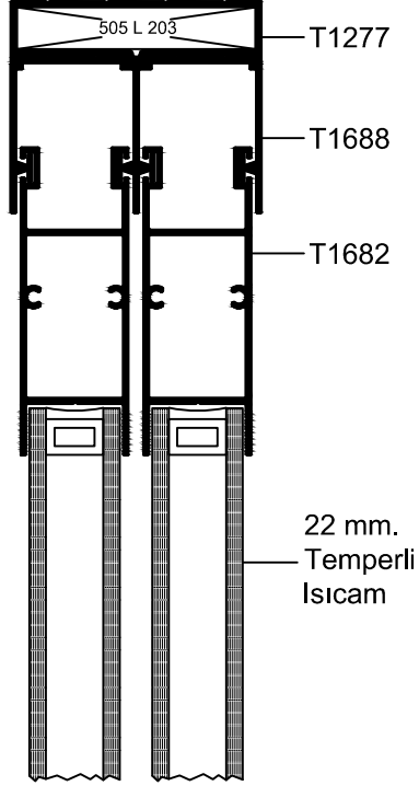
EŞİKSİZ SÜRME CAM BALKON
