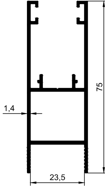
T1274 -0.865 kg/m
