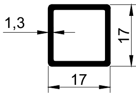
T-149 - 0,235 Kg/m
