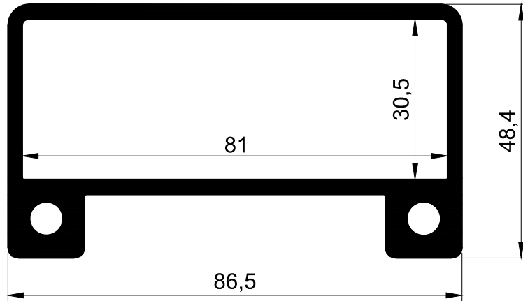
T-880A - 2,580 Kg/m 30*80 duvar flanşı
