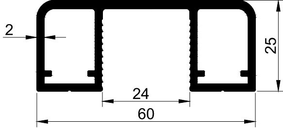
T-664 - 1,010 Kg/m 10+10mm. lamine cama göre
