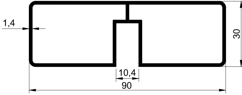
T-766 - 1.032 kg/m 4+4 mm. lamine cama göre
