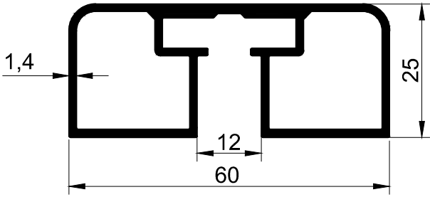
T-881 - 0,883 Kg/m 5+5 mm. lamine cama göre
