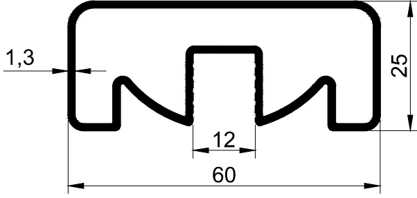
T-842 - 0,755 Kg/m
