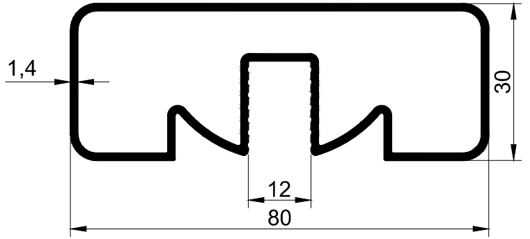
T-881B - 1,010 Kg/m 5+5 mm. lamine cama göre
