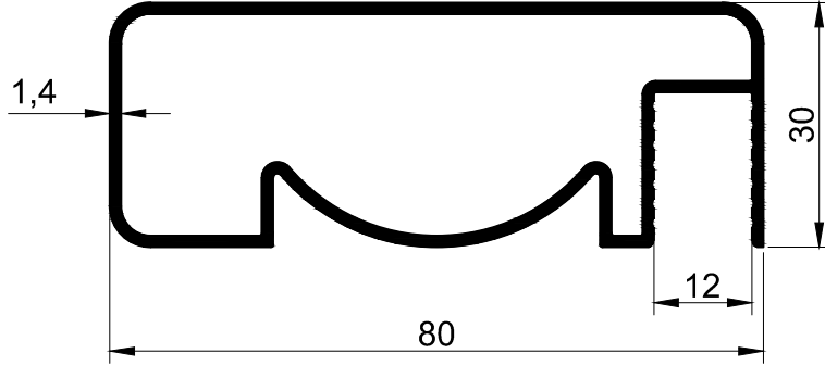
T-881C - 0,955 Kg/m 5+5 mm. lamine cama göre
