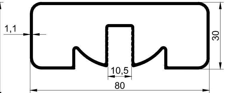
T-881B-1.1 - 0,800 Kg/m 4+4 mm. lamine cama göre
