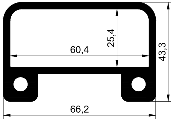
T-880 - 2,170 Kg/m 25*60 duvar flanşı
