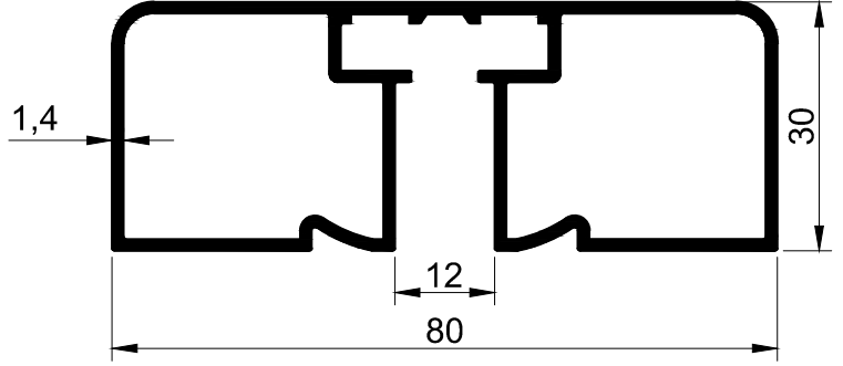
T-881A - 1,067 Kg/m 5+5 mm. lamine cama göre
