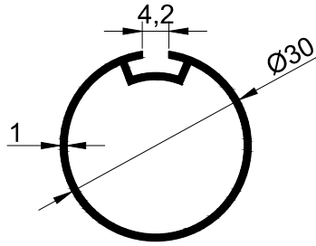
T 2148 - 0.285 kg/m
