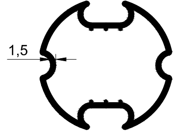
T 1121 - 0.621 kg/m
