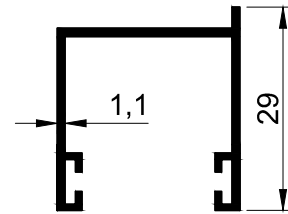
T 102 - 0.275 kg/m
