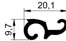
T 2131 - 0.191 kg/m
