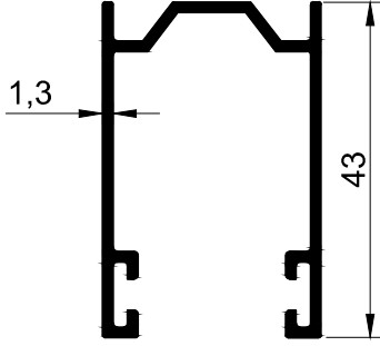
T 803 - 0.496 kg/m
