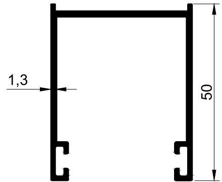
T 802 - 0.690 kg/m
