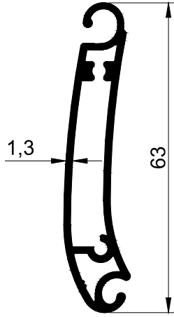
T 2130 - 0.598 kg/m
