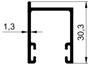
T 817 - 0.334 kg/m
