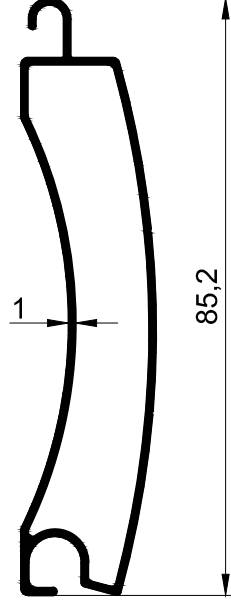
T 811 - 0.561 kg/m
