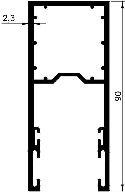
T 804 - 1.632 kg/m
