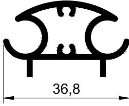
T 1120 - 0.507 kg/m
