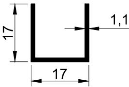
T 450 - 0.156 kg/m
