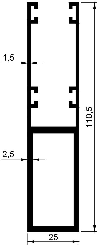
T 2139 - 1.630 kg/m
