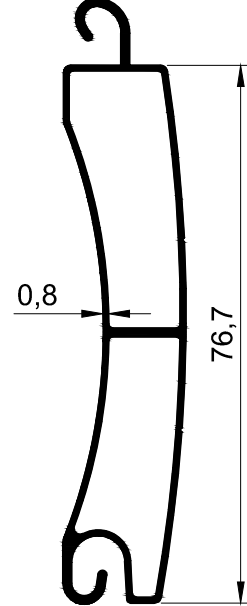
T 818 - 0.540 kg/m
