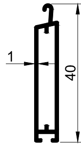
T 814 - 0.258 kg/m
