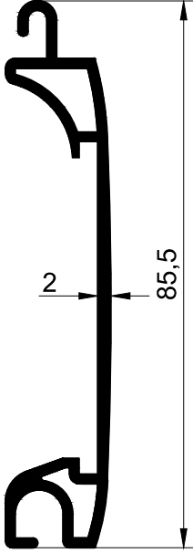
T 812 - 0.766 kg/m
