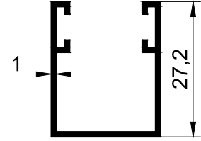
T 1133 - 0.250 kg/m
