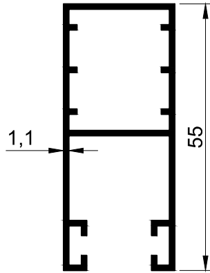
T 813 - 0.560 kg/m
