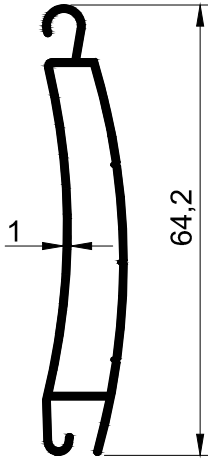
T 810 - 0.410 kg/m
