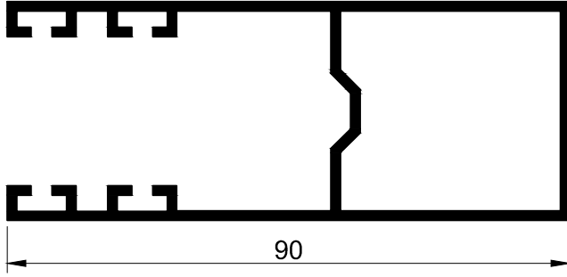
T 2133 - 1.220 kg/m
