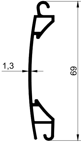
T 809 - 0.464 kg/m
