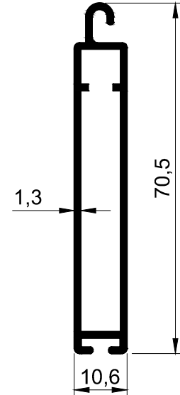
T 2135 - 0.578 kg/m
