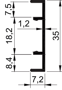
T601 - 0.180 kg/mt
