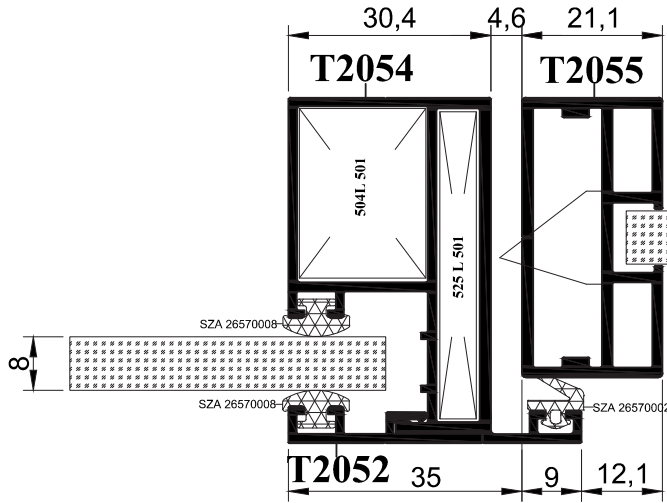
B DETAYI
