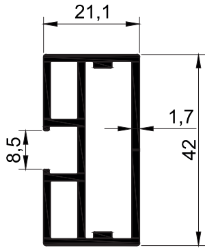
T2055 - 0.720 kg/mt
