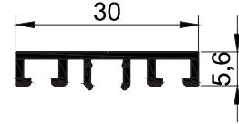
T2048 - 0.195 kg/mt
