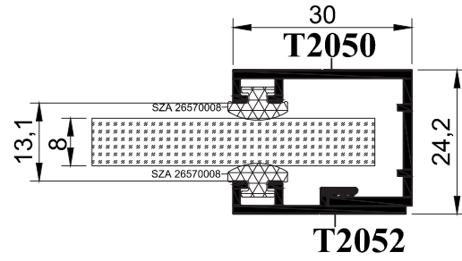
D DETAYI
