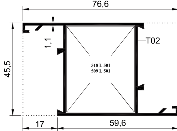
A45 Z 02 -1.1mm.-0.680 kg/mt
