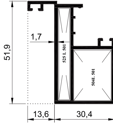
T2054 - 0.865 kg/mt
