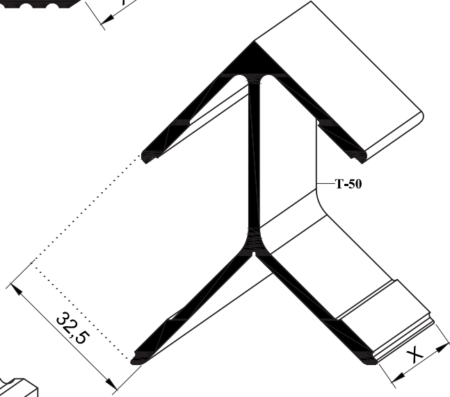
T518 - 1.230 kg/mt
