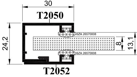
A DETAYI
