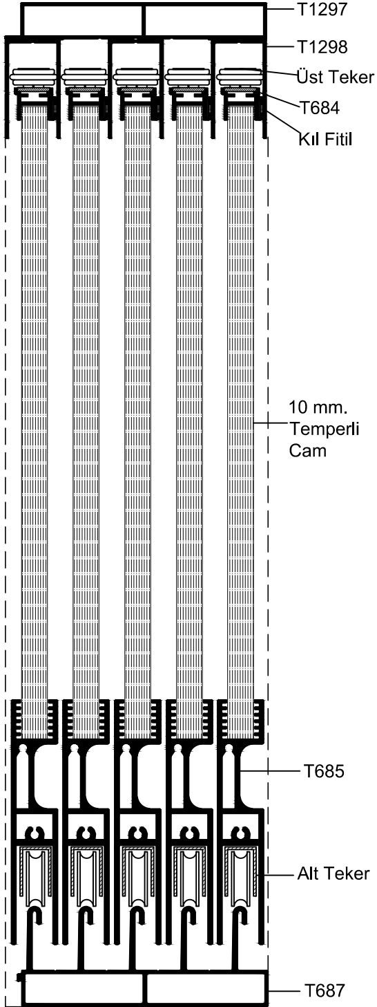
EŞİKLİ SİSTEM SÜRME CAM BALKON
