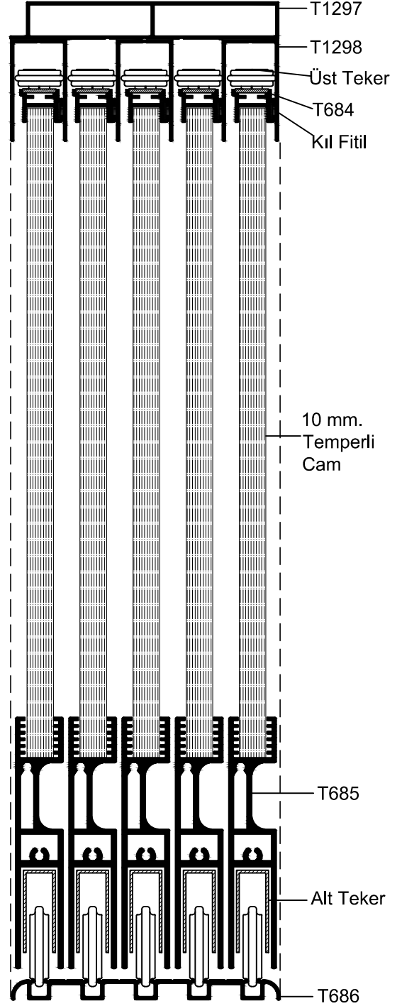
EŞİKSİZ SİSTEM SÜRME CAM BALKON
