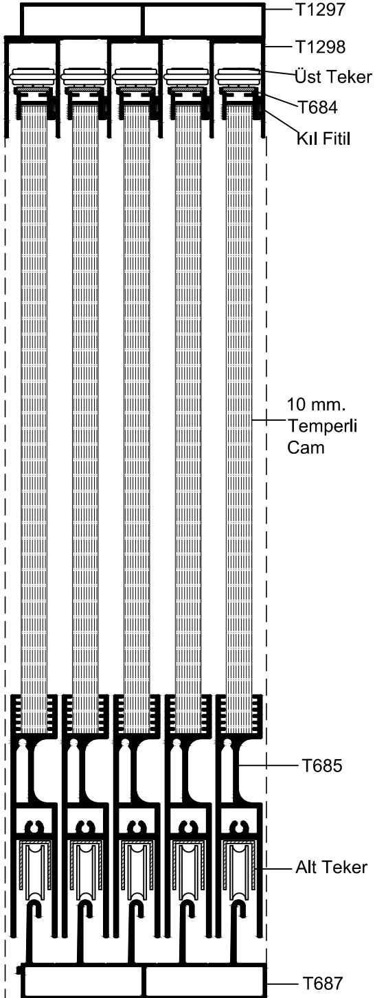
EŞİKLİ SİSTEM SÜRME CAM BALKON
