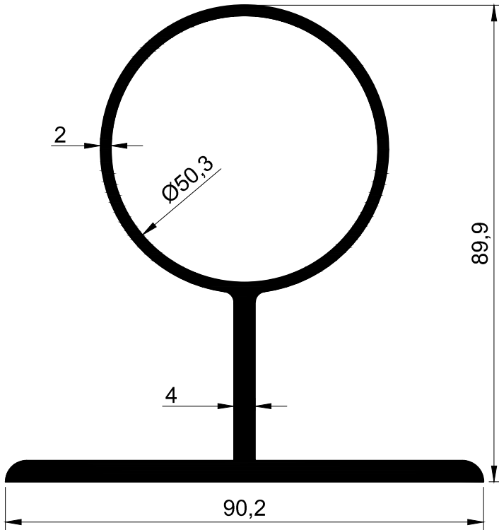
T-1188 - 2.195 kg/m
