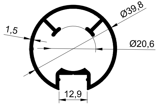
T-2599 - 0.665 kg/m
