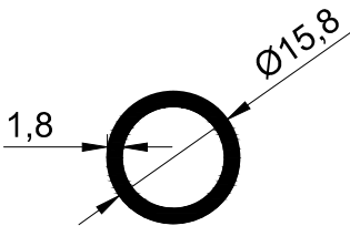
T430-1.8 - 0.215 kg/m
