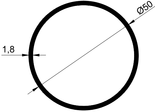
T427-1.8 - 0.745 kg/m
