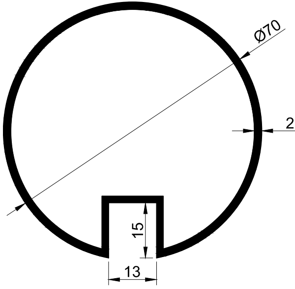
T-2391 - 1.233 kg/m
