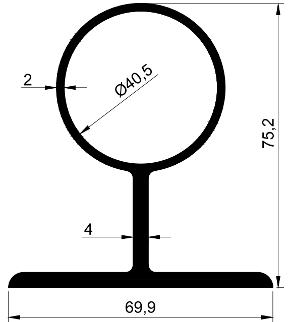
T-1190 - 1.760 kg/m
