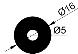
T-429 - 0.505 kg/m
