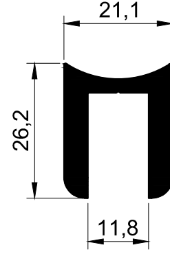
T-1191 - 0.710 kg/m
