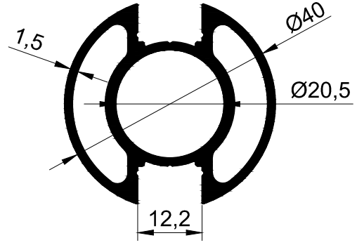
T-2154 - 0.950 kg/m
