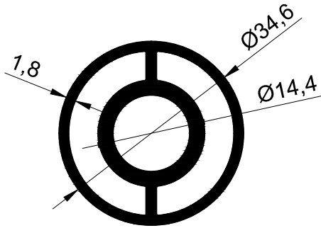
T-2181 - 0.985 kg/m
