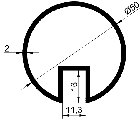
T-2531 - 0.925 kg/m
