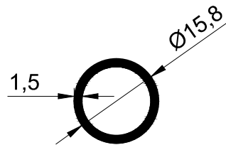
T430-1.5 - 0.191 kg/m
