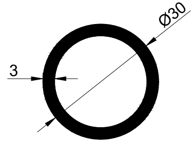
T435-3.0 - 0.694 kg/m
