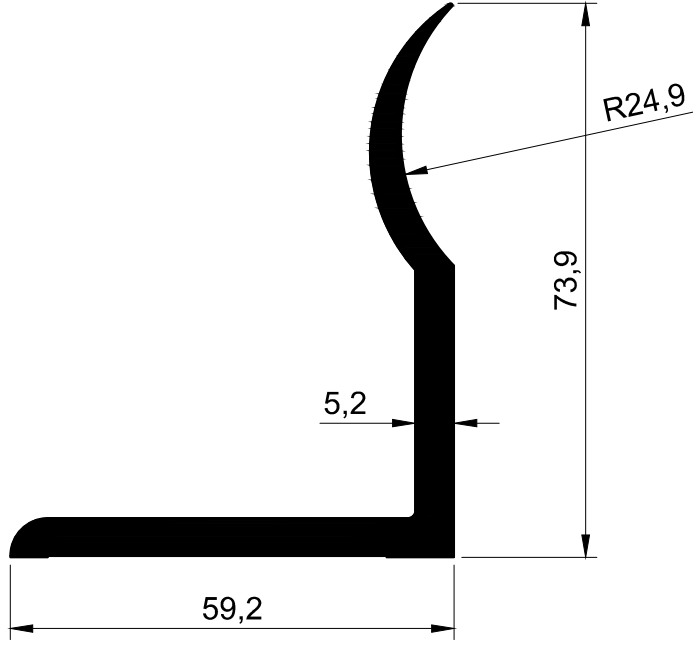
T-1189 - 1.640 kg/m
