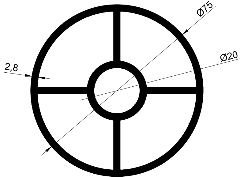
T-2182 - 2.975 kg/m
